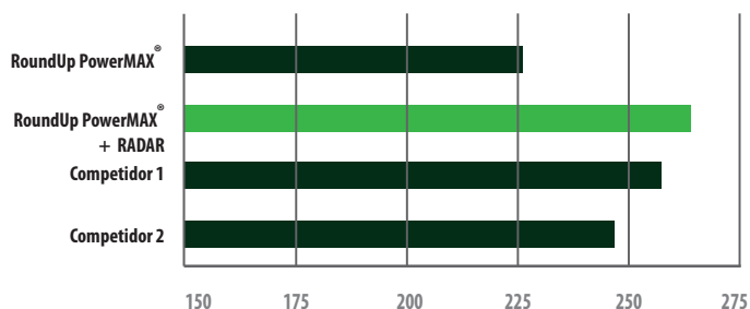
Prueba de atomización en túnel de viento • Dr. Greg Kruger, 1/2013 Universidad de Nebraska
